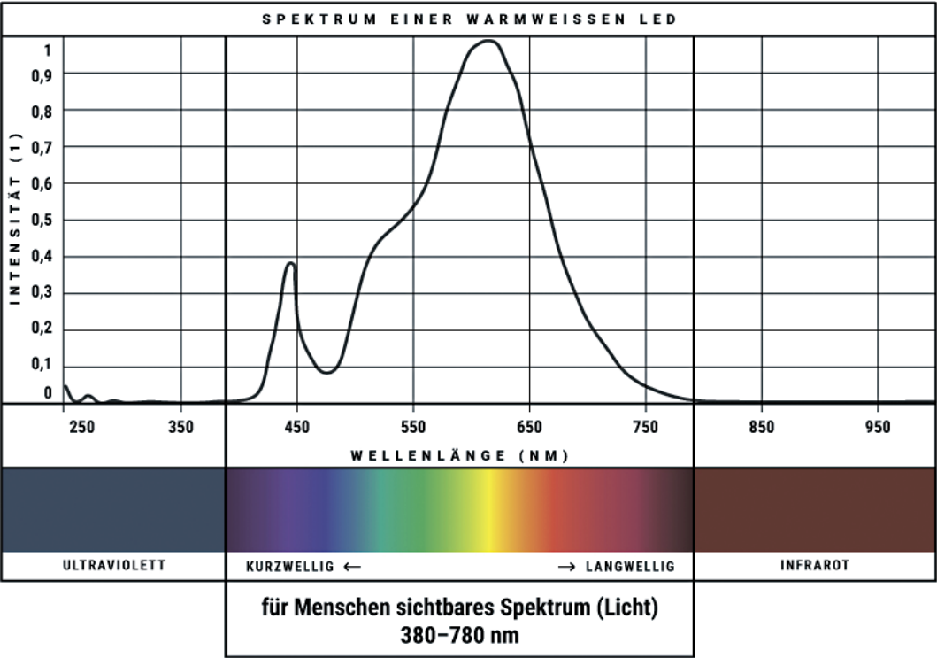
Abb. 10: Die Spektralkurve geht ins Detail und zeigt den emittierten Strahlungsanteil eines Leuchtmittels. © Illustration: Vandasye 2017.
